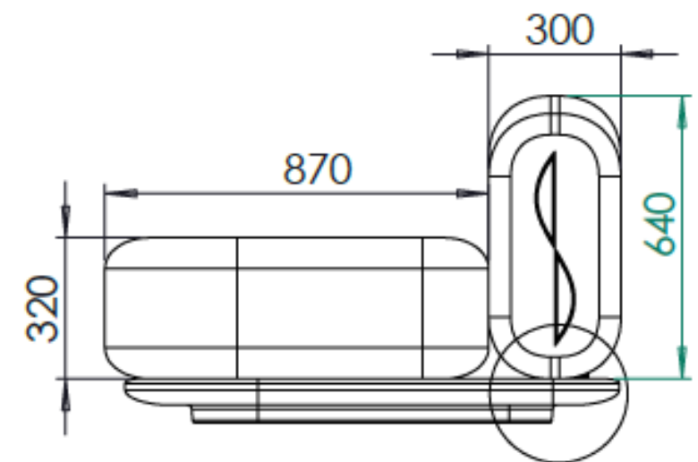
DETALHE A ESCALA 1 : 5
